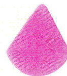
RHODAMINE B
